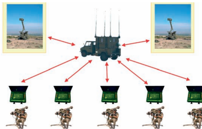
Composición del sistema COAAS de una unidad Mistral
