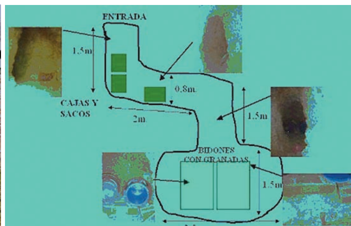
Croquis de un depósito de munición
